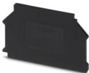
Концевая крышка, длина: 58 мм, ширина: 2,2 мм, высота: 35,05 мм, цвет: черный
