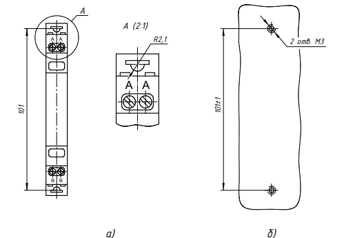
Рисунок Б.2 - Присоединительные размеры элементов крепления RC-модуля на монтажную панель (а) и разметка отверстий крепления на монтажной панели (б)
