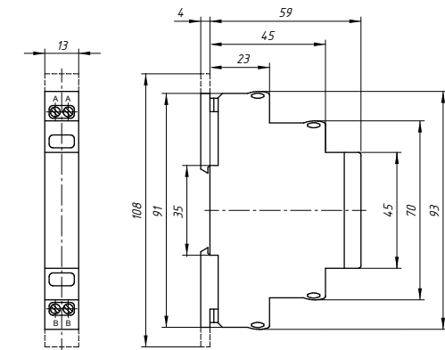
Рисунок Б.1 - Габаритные и присоединительные размеры RC-модуля
