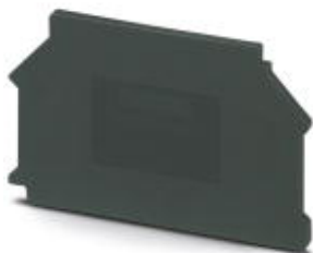
Крышка, длина: 58 мм, ширина: 2,2 мм, высота: 35,1 мм, цвет: темно-серая
