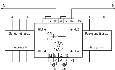
Рис. 1 - Схематичное изображение лицевой панели АВР МСВ
