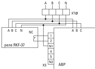
Рис. 2 - Схема подключения с применением реле контроля фаз
