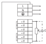
Рис 9. Схема подключения (MPS-200W-12, MPS-350W-12, MPS-500W-12)
