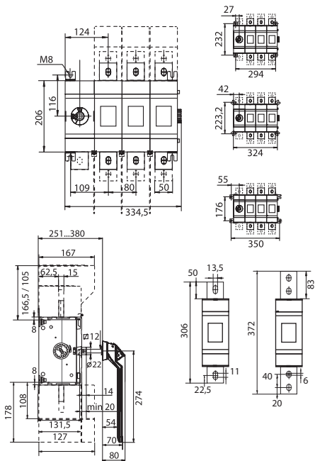
Рис. 8 – Габаритные и установочные размеры рубильников 1000-1600А 3Р
