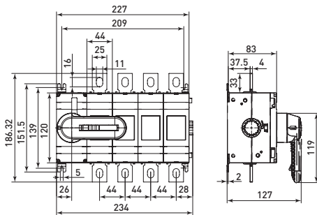
Рис. 6 – Габаритные и установочные размеры рубильников 315-400 А 4Р
