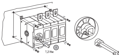
Рис. – 20 Монтаж моделей 40–125 А
