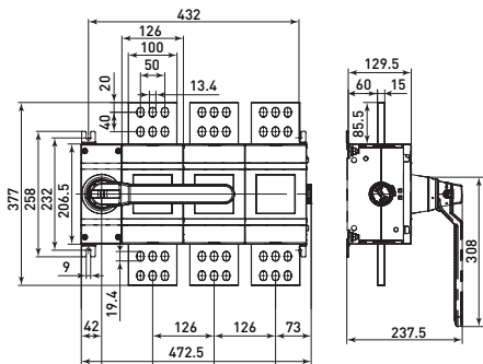
Рис. 11 – Габаритные и установочные размеры рубильников 2000-2500 А ЗР
