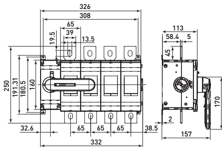
Рис. 9 – Габаритные и установочные размеры рубильников 630-800 А 4Р
