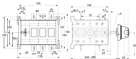
Рис. 13 – Габаритные и установочные размеры реверсивных рубильников 160-250 А 3Р
