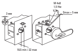
Рис. 24 – Установка рукоятки для управления через дверь
