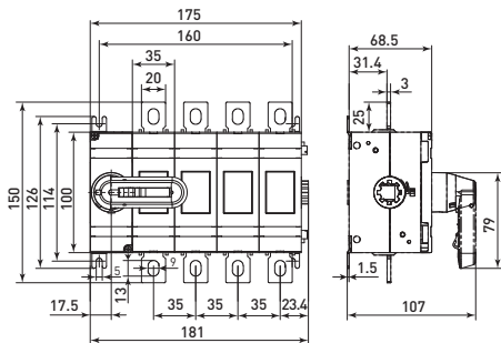
Рис. 5 – Габаритные и установочные размеры рубильников 160-250 А 4Р
