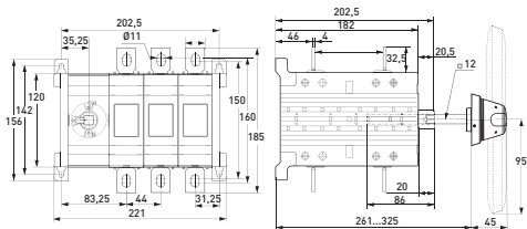
Рис. 15 – Габаритные и установочные размеры реверсивных рубильников 315-400 А 3Р
