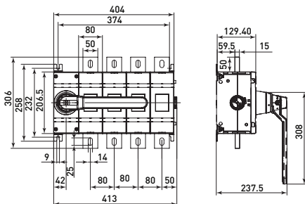
Рис. 10 – Габаритные и установочные размеры рубильников 1000-1600 А 4Р
