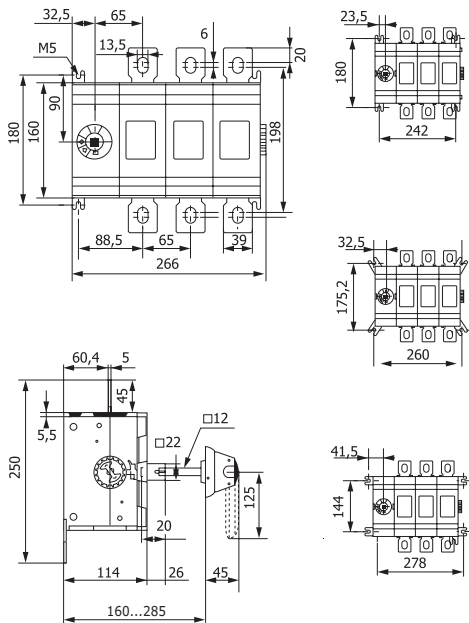
Рис. 7 – Габаритные и установочные размеры рубильников 630-800 А 3Р
