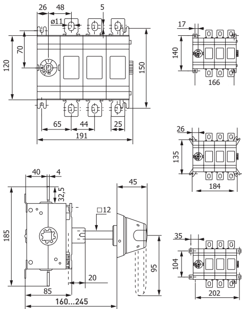
Рис. 4 – Габаритные и установочные размеры рубильников 315-400 А 3Р
