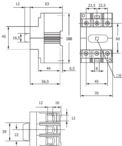
Рис. 1 – Габаритные и установочные размеры рубильников 40-125А 3Р
