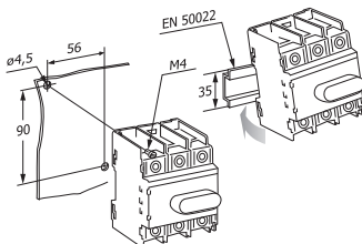
Рис. – 20 Монтаж моделей 40–125 А
