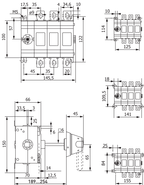
Рис. 3 – Габаритные и установочные размеры рубильников 160-250 А 3Р
