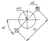
Рис.25 – Размеры выреза для ручки
