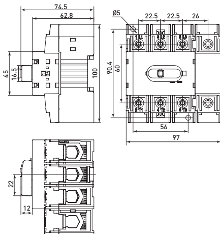
Рис. 2 – Габаритные и установочные размеры рубильников 63-125 А 4Р
