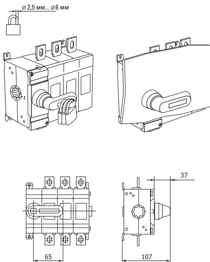
Рис. 22 – Установка рукоятки управления прямой установки 160-250 А
