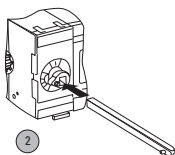
Рис. 21 – Установка переходника
