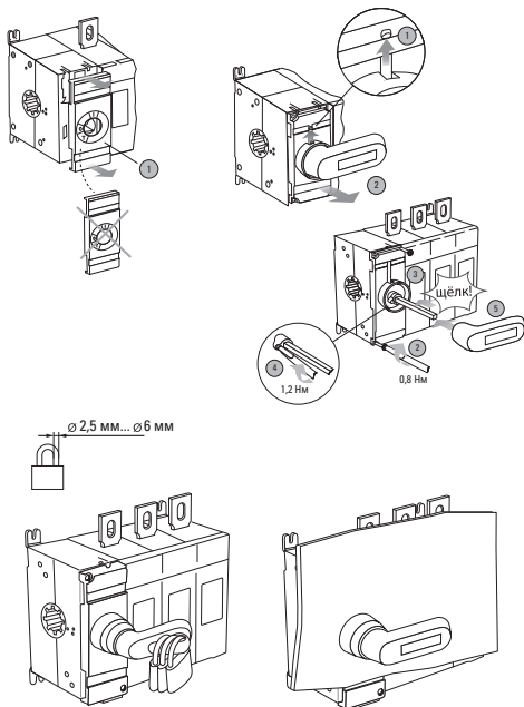
Рис. 23 – Установка рукоятки управления прямой установки 315-2500А
