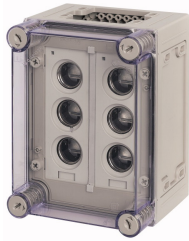
Блок предохранителей , 2х3хE33 , ВхШхД = 250х190х150 мм
