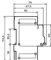
Рис. 4 – Габаритные размеры. Вар. 1
