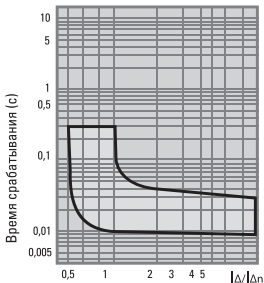
Рис. 1 – Время-токовые характеристики срабатывания дифференциальной защиты
