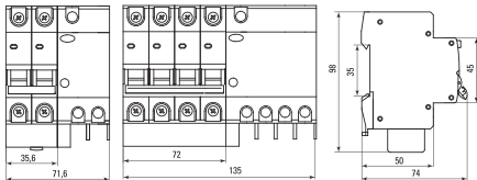
Рис. 5 – Габаритные размеры. Вар. 2
