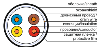
Рисунок 6 – Конструкция кабеля типа RS-485 нг(A) (количество жил 2×2) / Figure 6 – Cable design of RS-485 нг(A) type (amount of cores 2×2)
