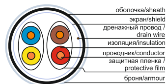
Рисунок 4 – Конструкция кабеля типа RS-485 КГнг(A) (количество жил 2×2) / Figure 4 – Cable design of RS-485 КГнг(A) type (amount of cores 2×2)
