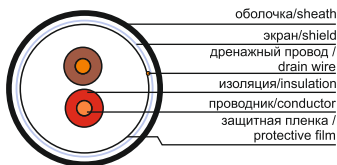
Рисунок 5 – Конструкция кабеля типа RS-485 нг(A) (количество жил 1×2) / Figure 5 – Cable design of RS-485 нг(A) type (amount of cores 1×2)
