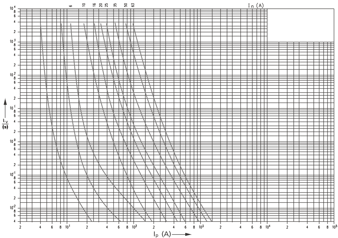
Zeit-/Stromkennlinie D01, D02, DII, DIII gG/gL
