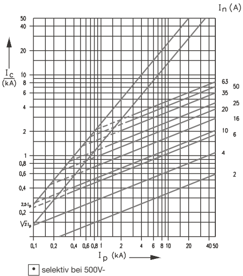
Strombegrenzungsdiagramm gG/gL 500V~ D01, D02, DII, DIII Sicherungseinsätze
