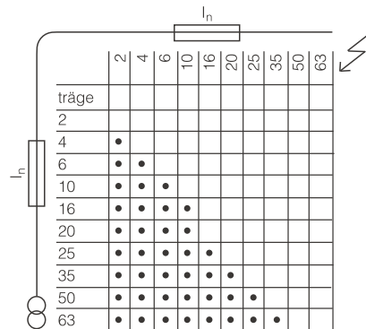
Selektivität gL/gL Sicherungen D01, D02, DII, DIII
