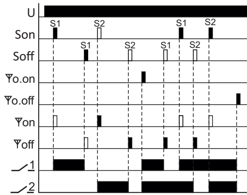
Диаграмма работы для режимов «ON» и «OFF»
