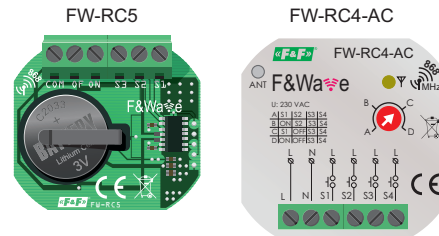
Встраиваемые под кнопочные выключатели: с автономным питанием и с сетевым 230В AC
