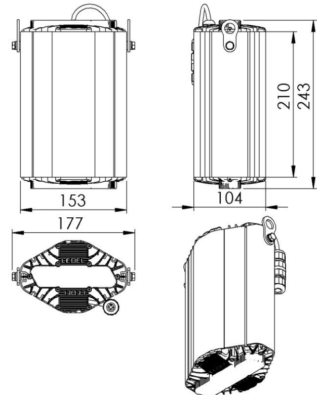
Рисунок 1 Светильник «L-lego II 55» Подвесное крепление.
