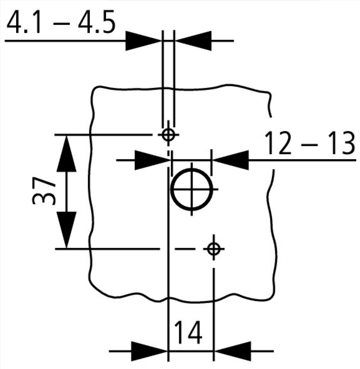
Шаблоны сверления для двери
