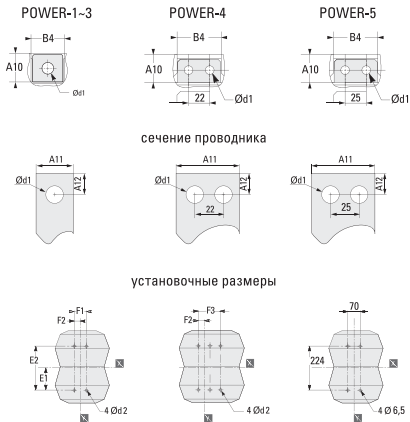
Рис. 4 - Присоединительные размеры
