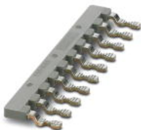
Гребенчатый мостик, 10 контактов, для клемм BK 4 на ленте
