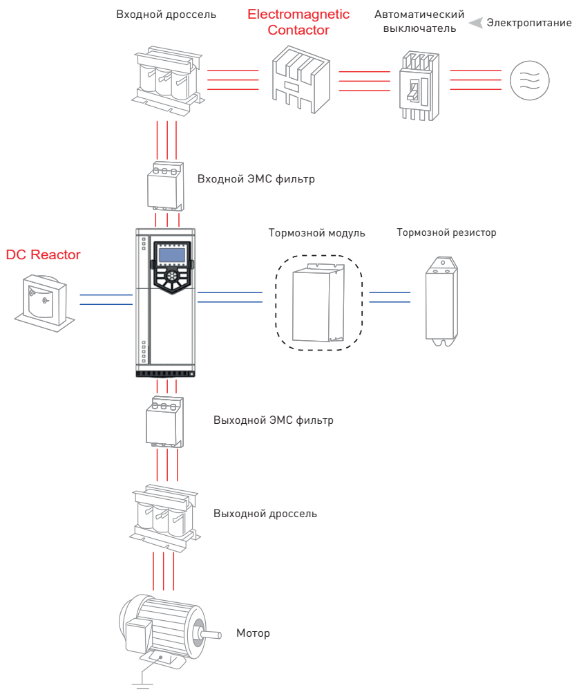
Рис. 5 - Упрощенная схема установки периферийных устройств
