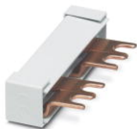
Монтажные перемычки для модуля с соединительным шагом 17,5 мм, 2-фазные, 4-полюсные
