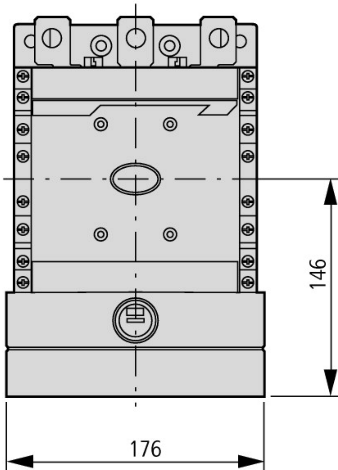
Силовые контакторы с перемычкой для соединения звездой и с крышкой для клемм для DILM500
