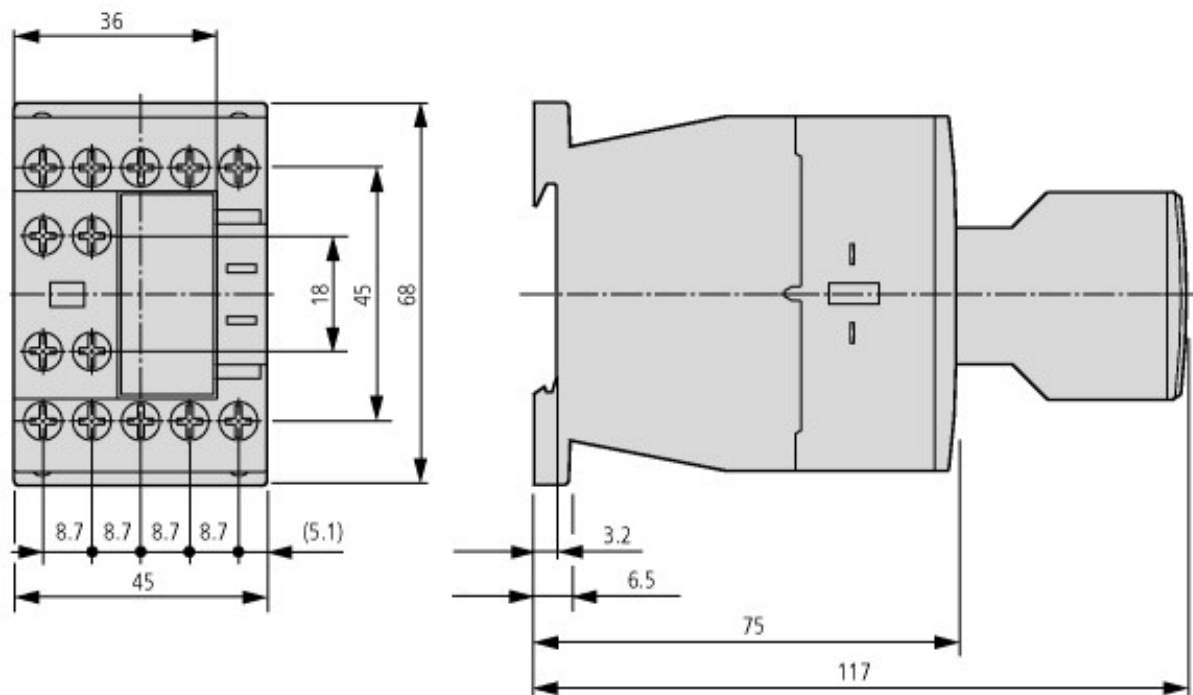
Силовой контактор со вспомогательным контактным модулем DILM32-XHI.../DILA-XHI...
