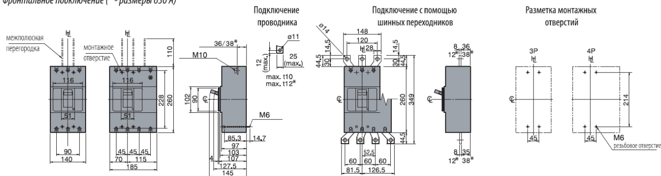
Фронтальное подключение (* - размеры 630 А)
