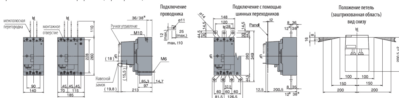
Фронтальное подключение с мотор-приводом (* - размеры 630 А)
