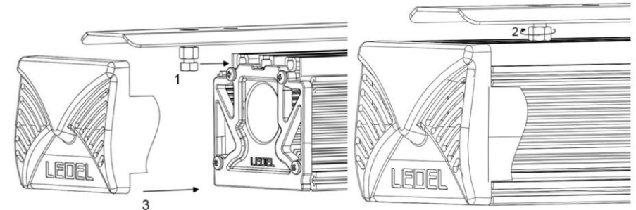
Рисунок 6 Схема монтажа подвесного крепления светильника
