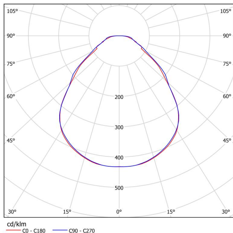
Рисунок 7 Тип КСС
