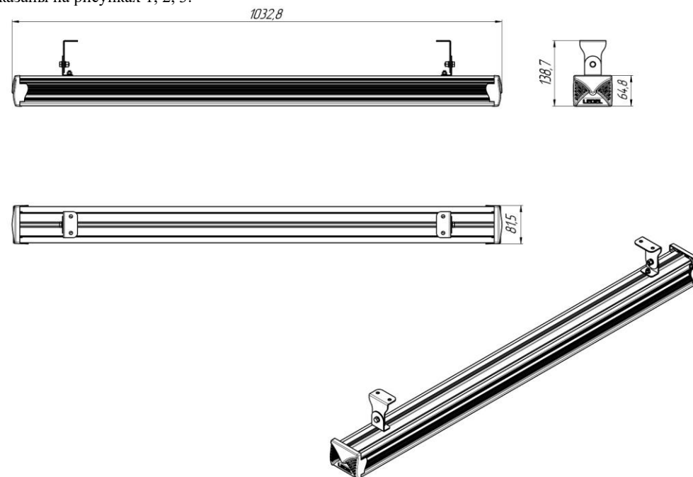
Рисунок 1 Светильник «L-industry NEW 48Т». Поворотный вариант
