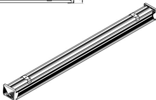
Рисунок 3 Светильник «L-industry NEW 48T». Задвижной вариант
