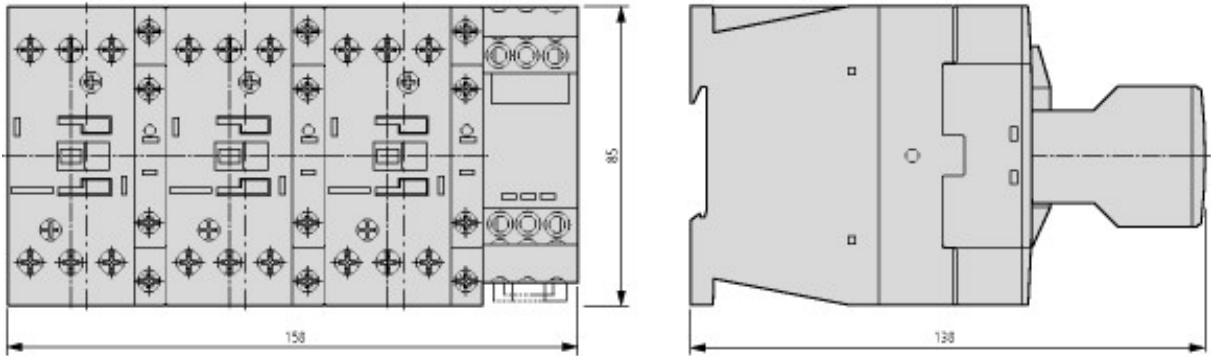
Базовое устройство с функциональным блоком вспомогательного контакта
