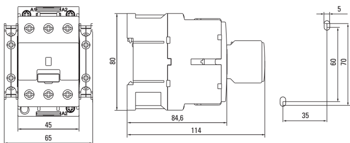
Рис. 5 – Габаритные и установочные размеры контакторов KMЭ 32A, KMЭ 38A
