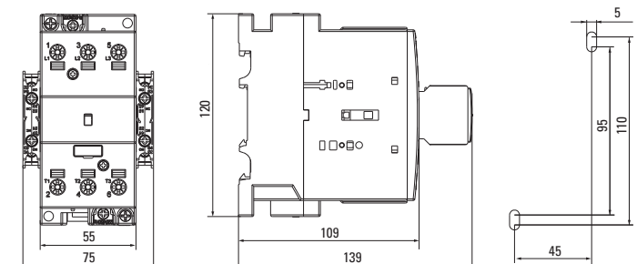
Рис. 6 – Габаритные и установочные размеры контакторов KMЭ 50A, KMЭ 60A, KMЭ 65A
