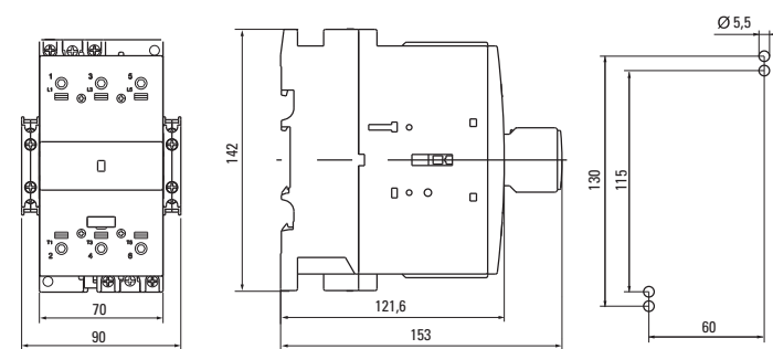
Рис. 7 – Габаритные и установочные размеры контакторов KMЭ 80A, KMЭ 90A, KMЭ 100A
