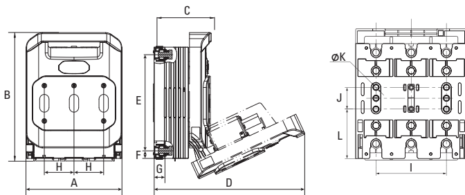
Рис. 2 - Габаритные размеры выключателя-разъединителя УБРЭ v2 250-630 А ЕКF
