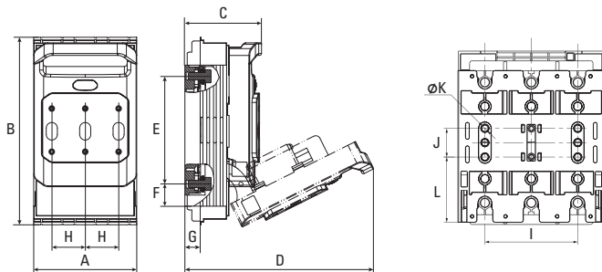
Рис. 1 - Габаритные размеры выключателя-разъединителя УБРЭ v2 160 А ЕКF
