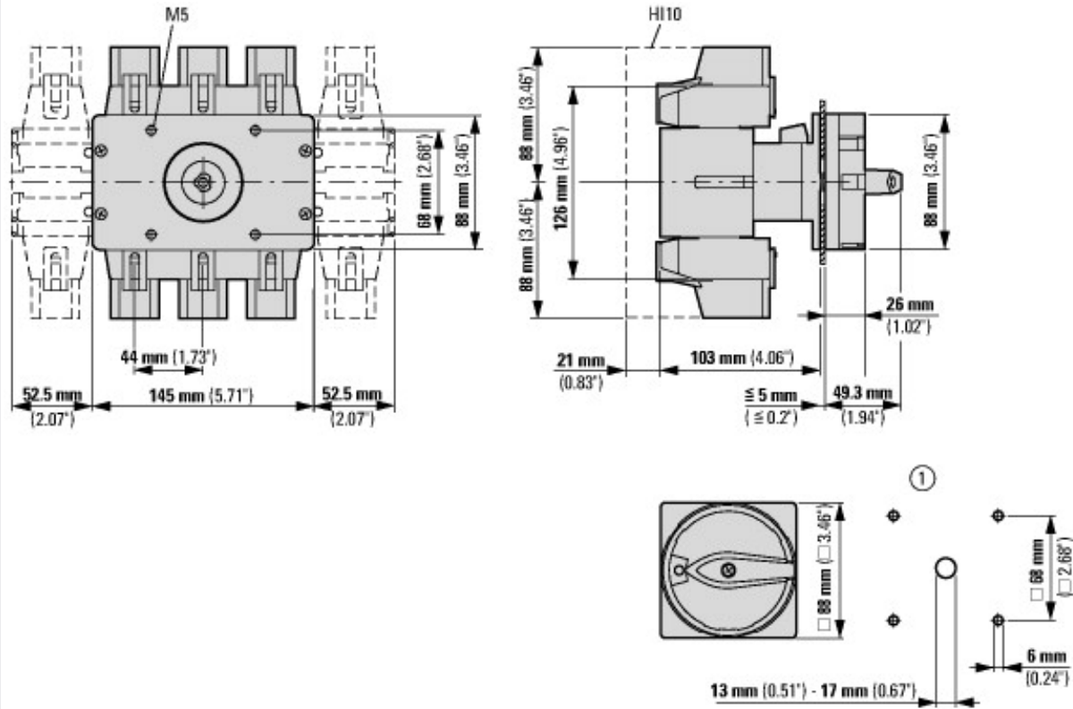
① Шаблоны сверления для двери
