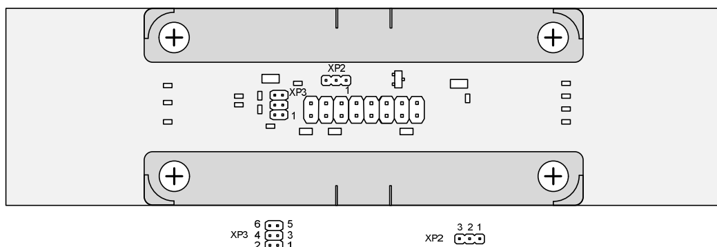
Рисунок 2 – Расположение перемычек XP2 и XP3
