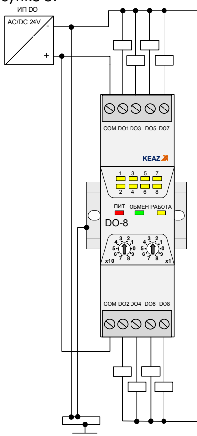
Рисунок 3 – Схемы подключения модуля
