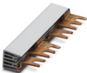
Монтажные перемычки для модуля с соединительным шагом 17,5 мм, 3-фазные, 6-полюсные
