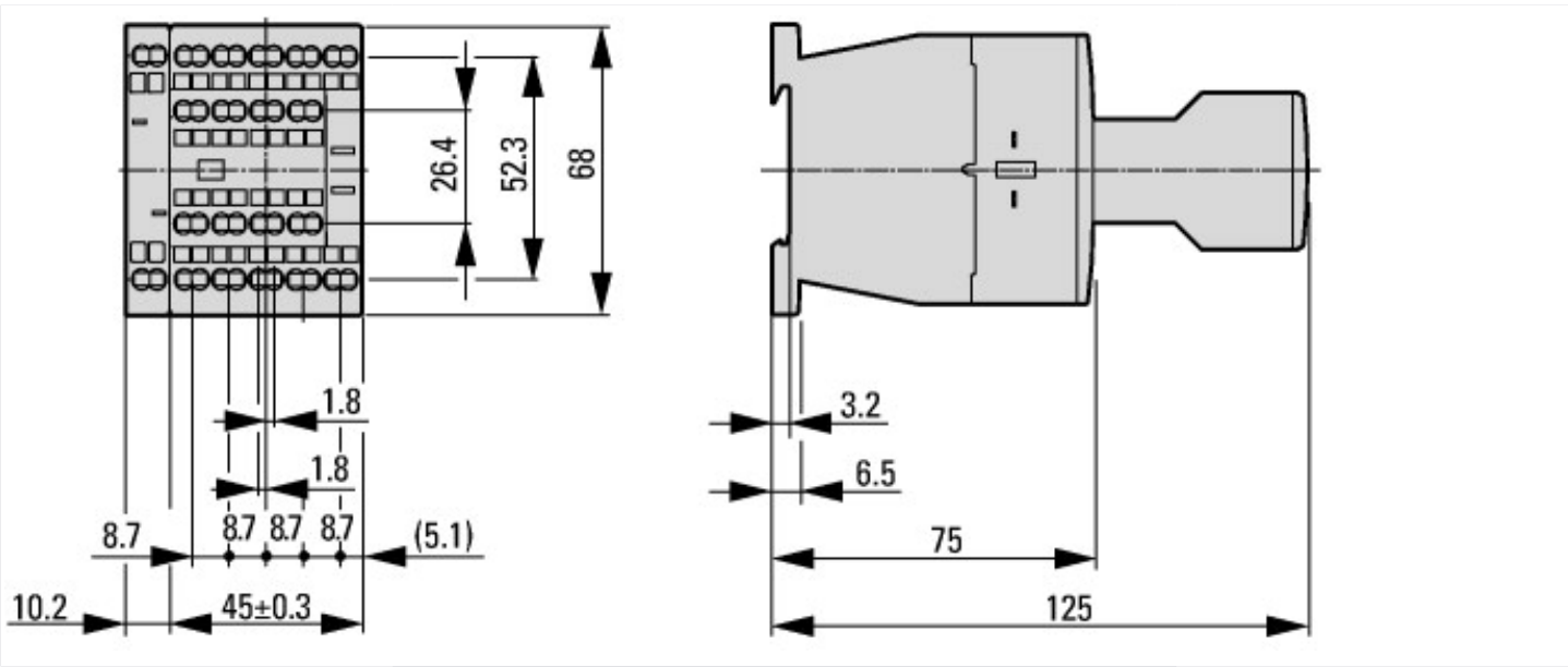
Силовой контактор со вспомогательным контактным модулем
