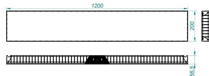
Рисунок 1б Светильник «L-school 32 Premium/Em», «L-school 55 Premium/Em»
