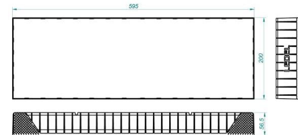
Рисунок 1а Светильники «L-school 16 Premium/Em»
