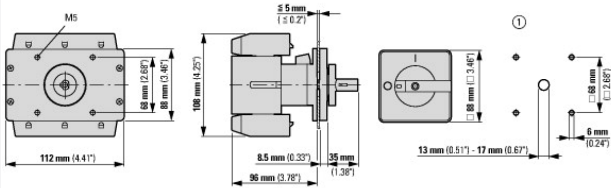
1 Шаблоны сверления для двери
