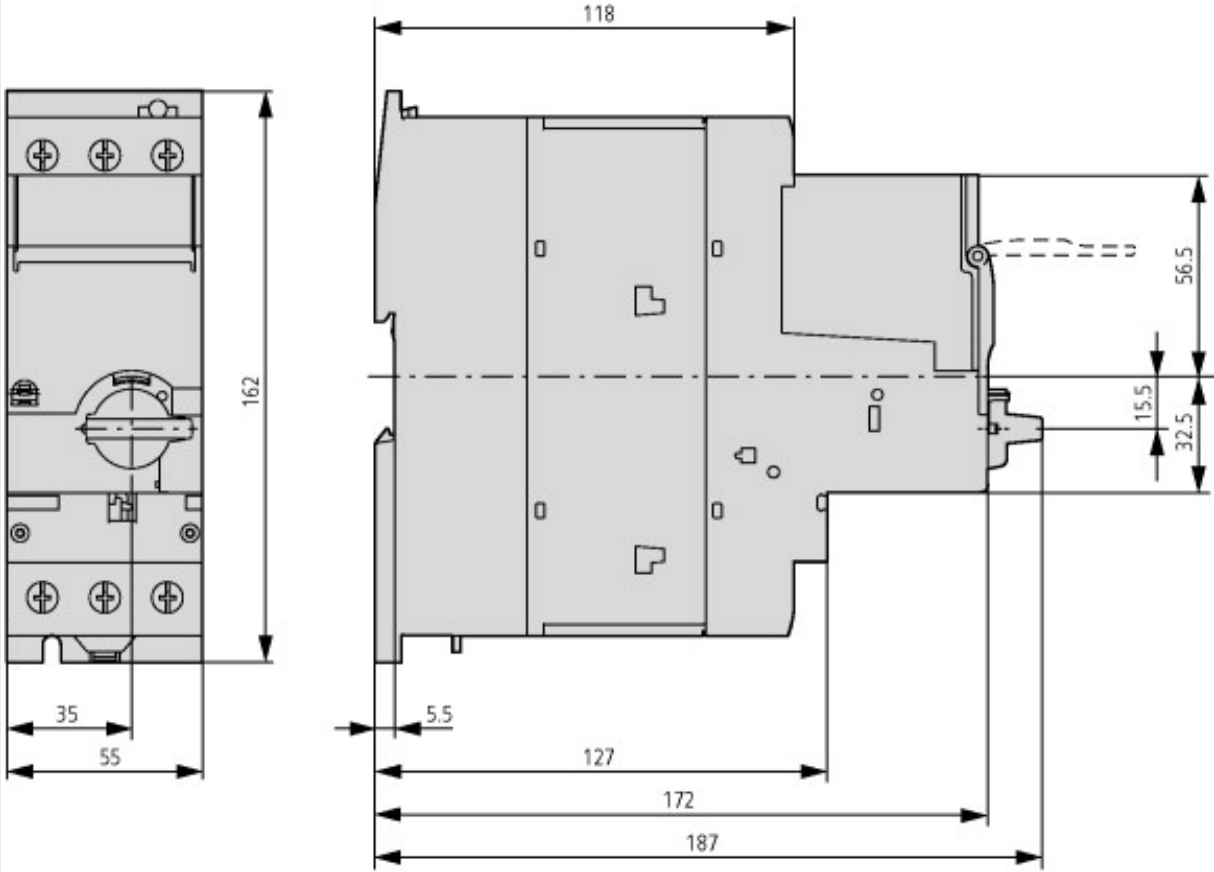
Основное устройство с расцепляющим модулем
