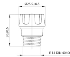
E 14 DIN 40400
