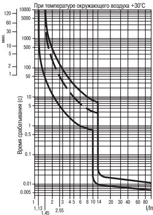
Рисунок 3. Характеристика D
