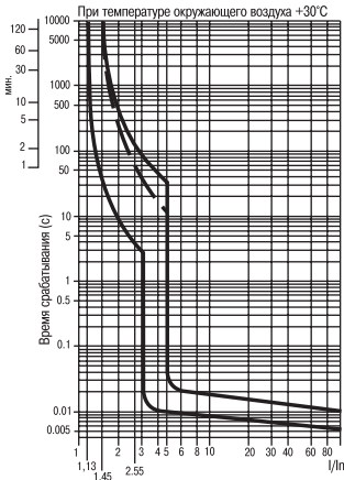
Рисунок 1. Характеристика В
