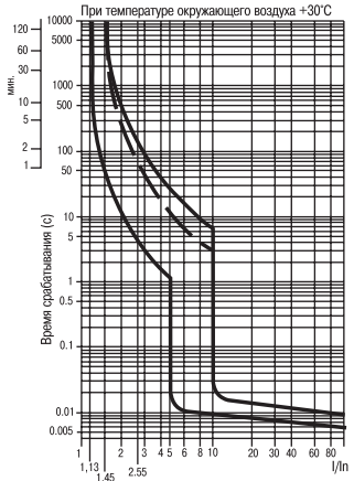
Рисунок 2. Характеристика С
