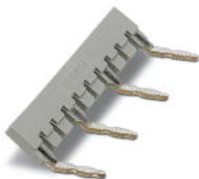
Гребенчатый мостик, размер шага: 6 мм, полюсов: 10, расположение полюсов: 1,4,7,10, цвет: серый
