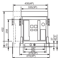
Вырез под рамку
