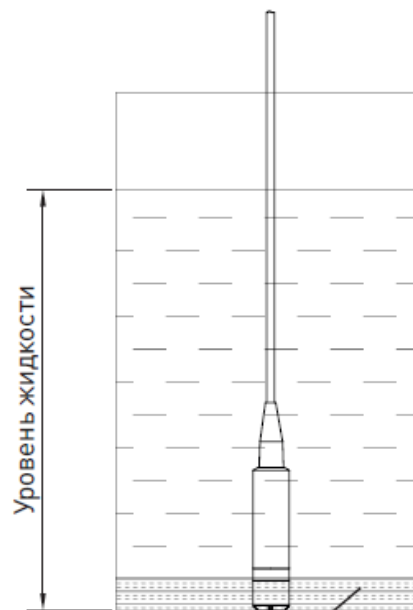
Глубина нечувствительности датчика ~25 мм
