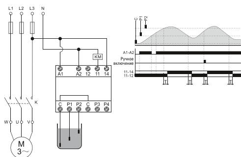
Одна емкость. Осушение по 2 датчикам
