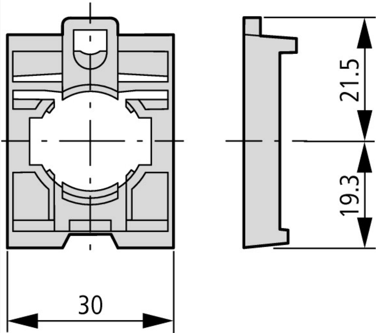
Крепёжный адаптер Крепежный адаптер (фронтальная установка) для 3 контактных/светодиодных индикаторов
