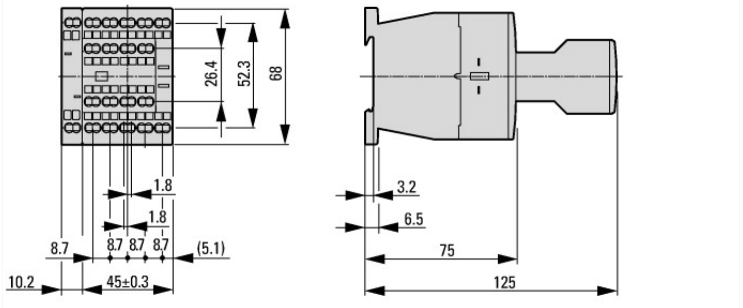
Силовые контакторы со вспомогательным контактным модулем
