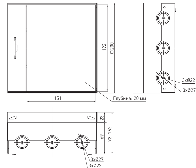
Рис. 1– Лючок металлический C-Line 6 (арт. cl-lnm-6)
