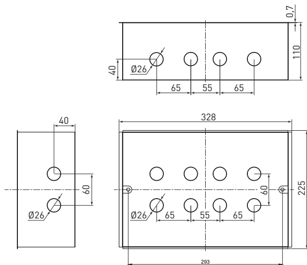
Рис. 7 – Напольная коробка под лючок C-Line 16-24 (cl-kl-n-k-16-24)
