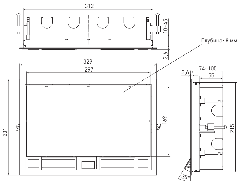
Рис. 6 – Лючок напольный с изменяемой глубиной C-Line 12 (арт. cl-ln-k-12 & cl-ln-k-12-1)
