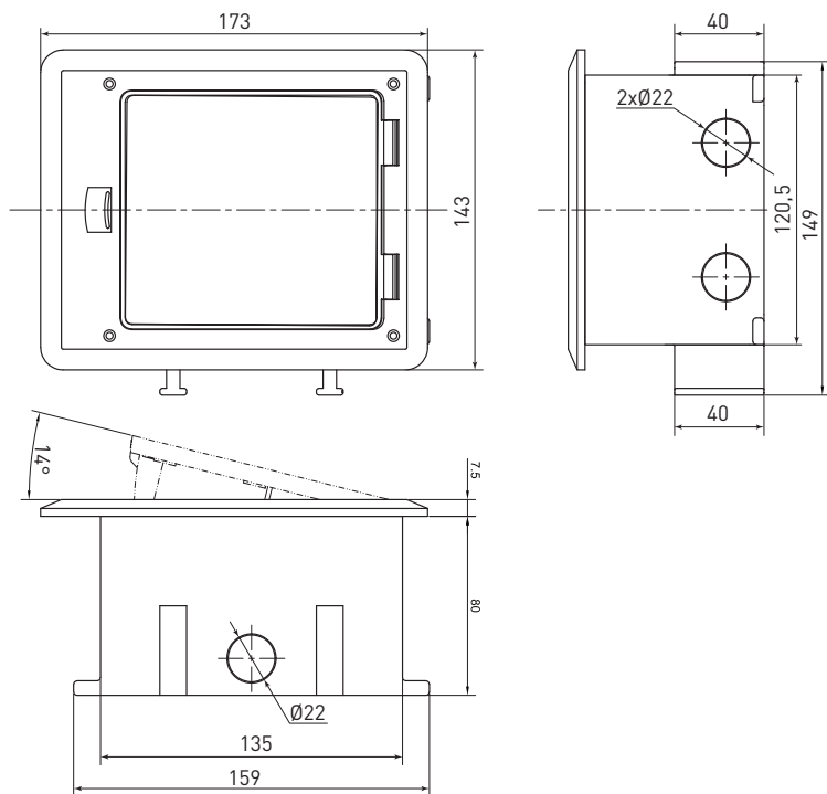
Рис. 3 – Лючок напольный IP66 C-Line WP-6 (арт. cl-lnwp-6)
