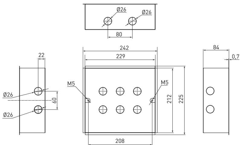
Рис. 4– Напольная коробка под лючок C-Line 12 (арт. cl-klп-k-12)
