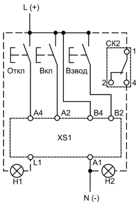
Рисунок 4 – Схема подключения привода с дистанционным взводом пружины включения, в том числе после аварийного отключения выключателя
