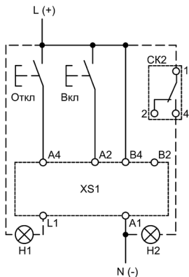
Рисунок 5 – Схема подключения привода с ручным взводом пружины включения
