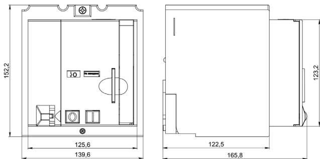
Рисунок 6 – Габаритные и установочные размеры привода
