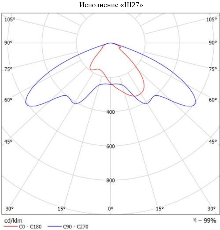
Рисунок 3 Типы КСС
