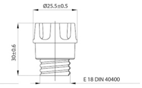
E 18 DIN 40400
