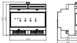
Рисунок 1. Габаритные размеры
