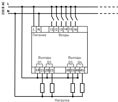
Рисунок 3. Схема подключения
