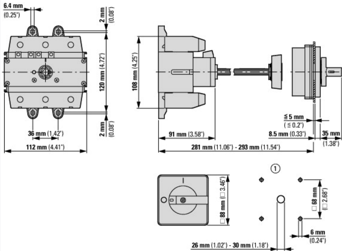
1 Шаблоны сверления для двери
