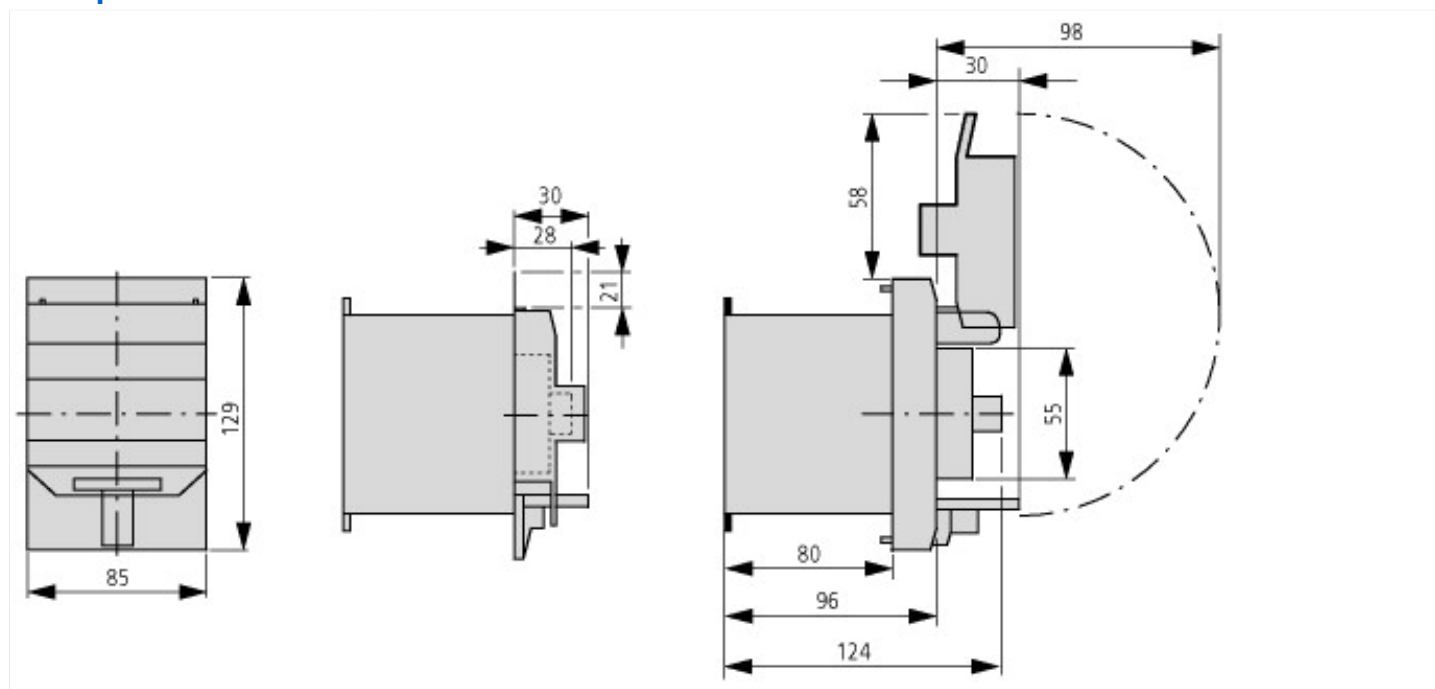
Изолированный корпус для монтажа
