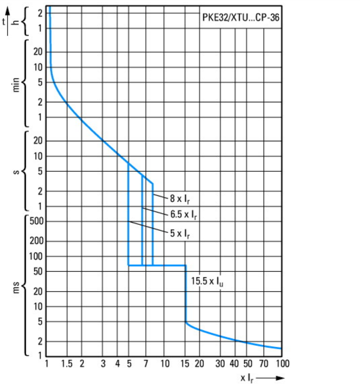
Характеристики расцепления
