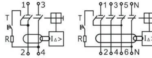
Рисунок В.1 - Принципиальные электрические схемы ВДТ
