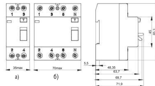
Рисунок Б.2 - Габаритные, установочные и присоединительные размеры ВДТ на номинальные токи 80-100А а) двухполюсного; б) четырехполюсного.
