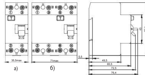
Рисунок Б.1 - Габаритные, установочные и присоединительные размеры ВДТ на номинальные токи 25-63А а) двухполюсного; б) четырехполюсного.
