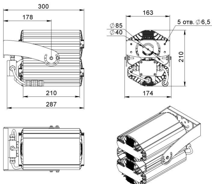
Рисунок 2 Светильник «L-lego II 110 banner» Поворотное крепление
