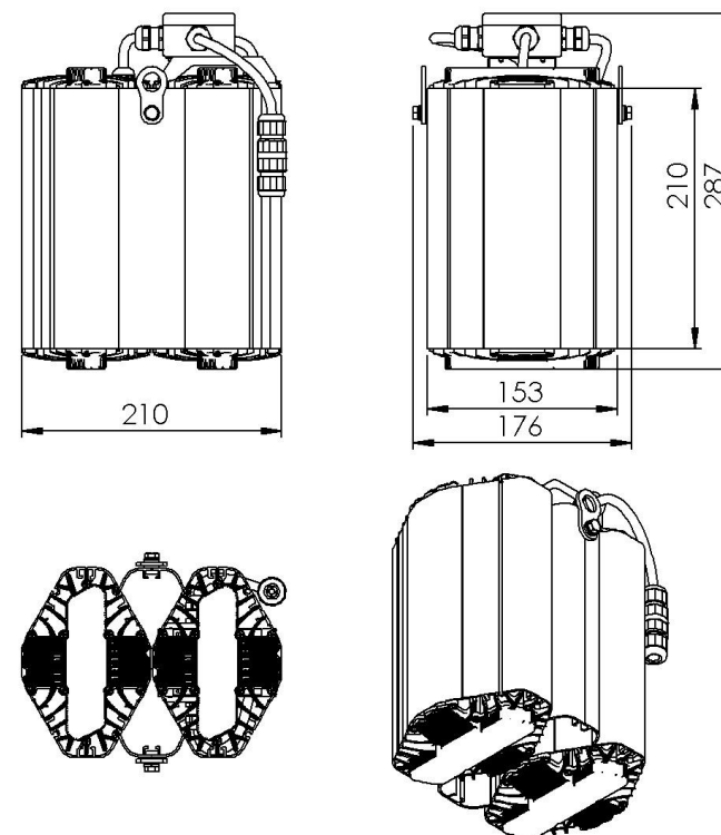
Рисунок. 1 Светильник «L-lego II 110» Подвесное крепление
