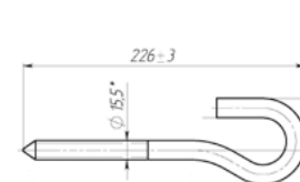
Крюк с резьбой BT16
