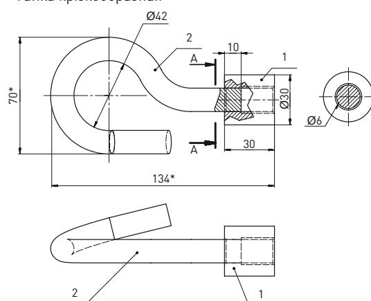
Крюк для плоской поверхности GHP16
